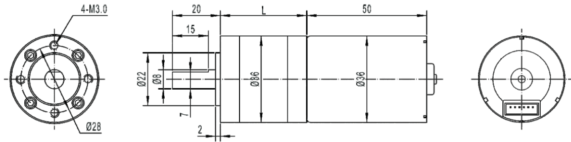
外形尺寸/Appearance dimension(mm)
